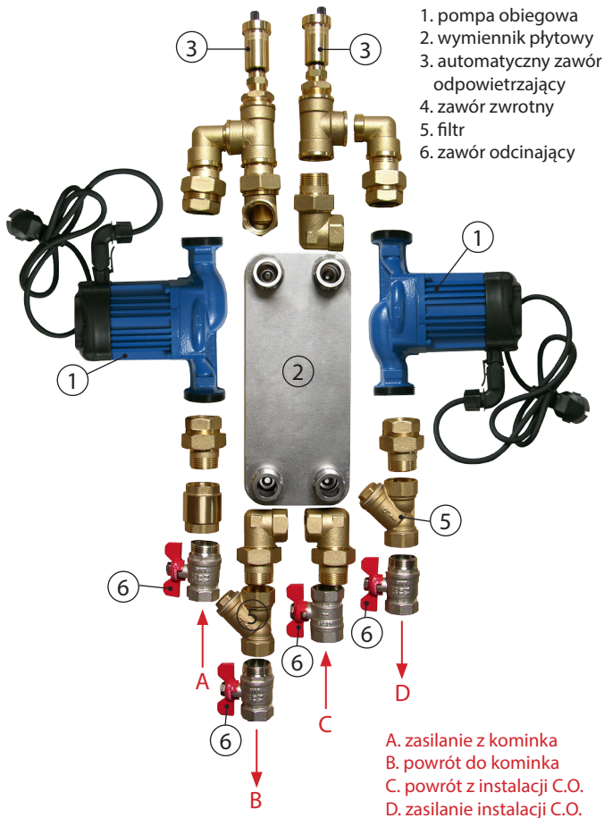
Rysunek 1. Schemat budowy zestawu mosiężnego wymiennikowo- płytowego.
